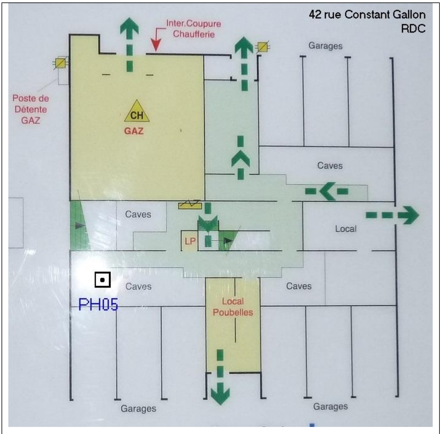
Planche (croquis) de repérage technique effectué par le cabinet : Cabinet AVICEA, auteur : LEVITAN Serge Dossier n° 2014-01-018 SL OPH77 - 42 du Adresse du bien : 42 rue Constant Gallon 77310 SAINT-FARGEAU-PONTHIERRY
